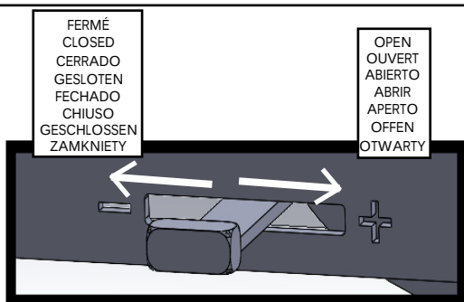
SECONDARY DRAUGHT / TIRAGE SECONDAIRE TIRO SECONDARIO / SECUNDAIR INLAAT ENTRADA DE AR SECUNDÁRIO / TIRAGGIO SECONDARIO SEKUNDÄRLUFT / CIAG WTORNY
