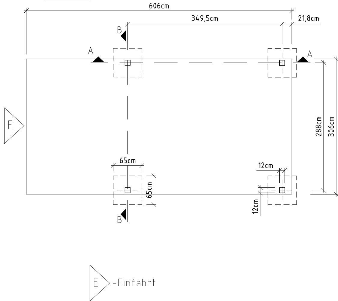
Grundriss
