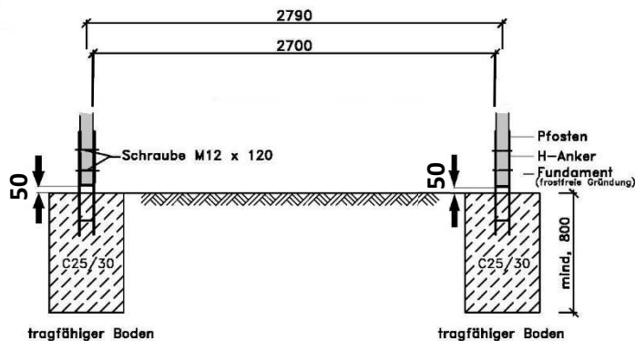
Schnitt C-C
