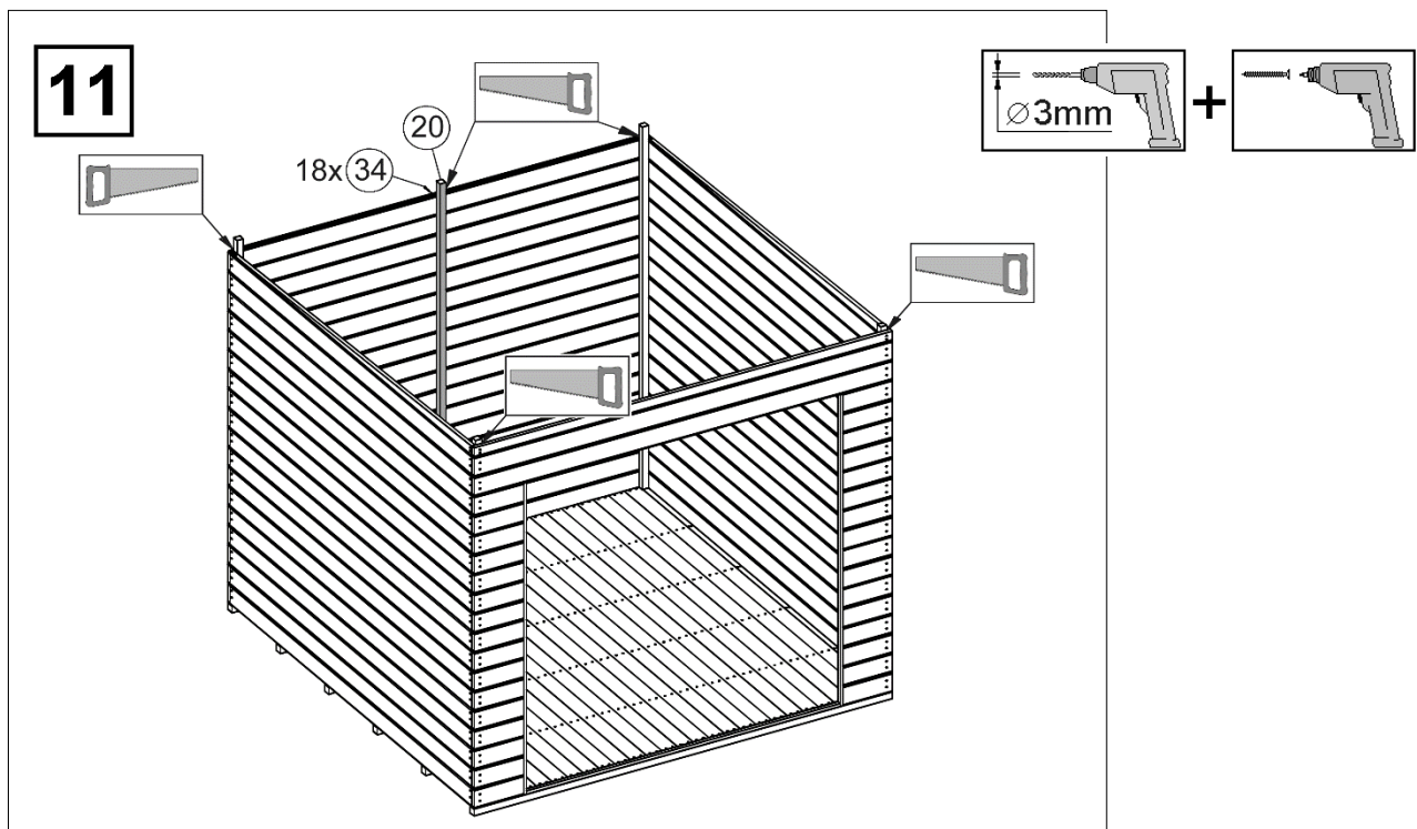
Abbildung Art.-Nr.: 227.2424.10400
