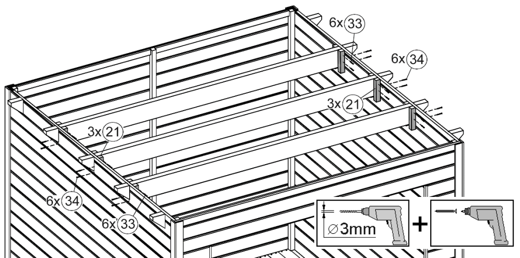
Abbildung Art.-Nr.: 227.2424.10400
