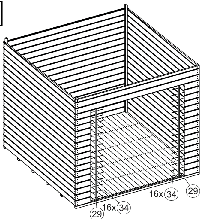
Abbildung Art.-Nr.: 227.2424.10400
