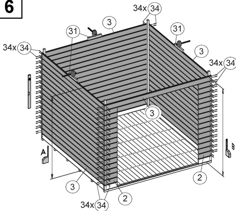
Abbildung Art.-Nr.: 227.2424.10400
