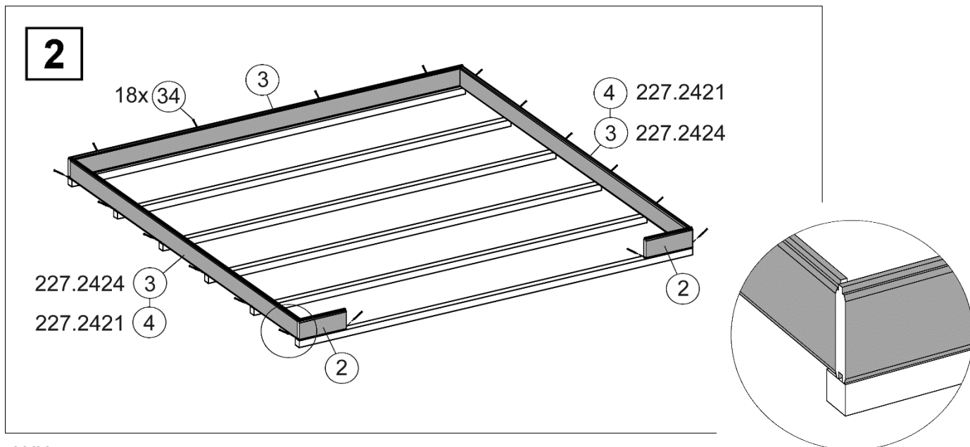
Abbildung Art.-Nr.: 227.2424.10400
