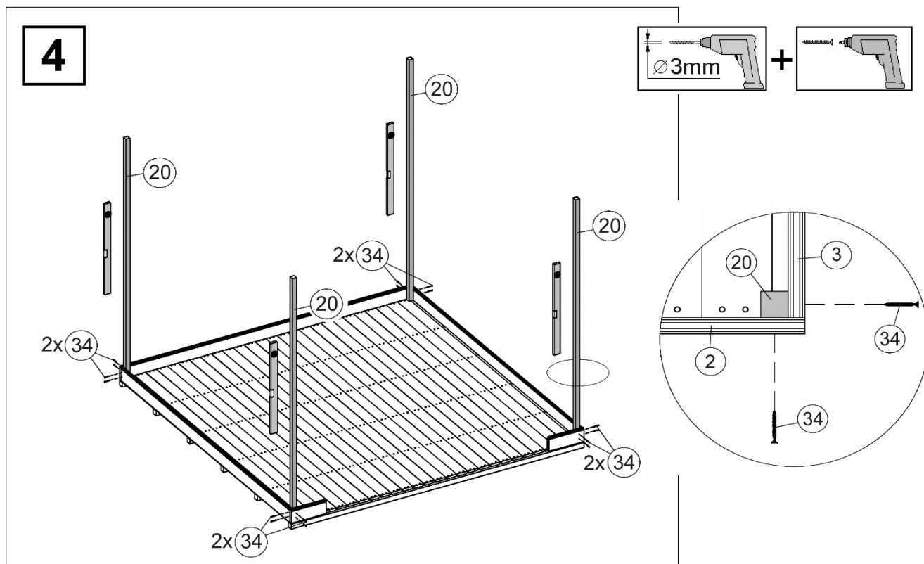
Abbildung Art.-Nr.: 227.2424.10400
