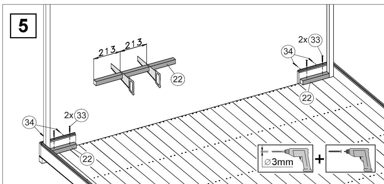
Abbildung Art.-Nr.: 227.2424.10400
