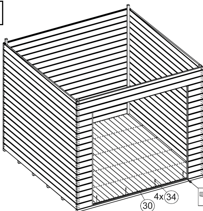
Abbildung Art.-Nr.: 227.2424.10400
