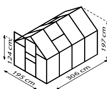
CALYPSO 5800
