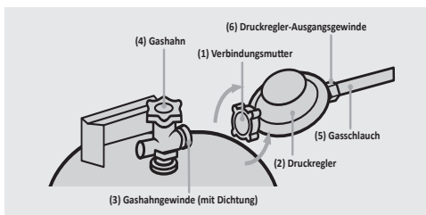
Abb.2: Montage des Druckreglers
