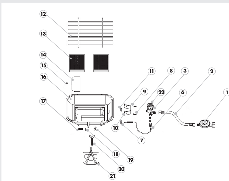
Abb. 4: Explosionszeichnung
