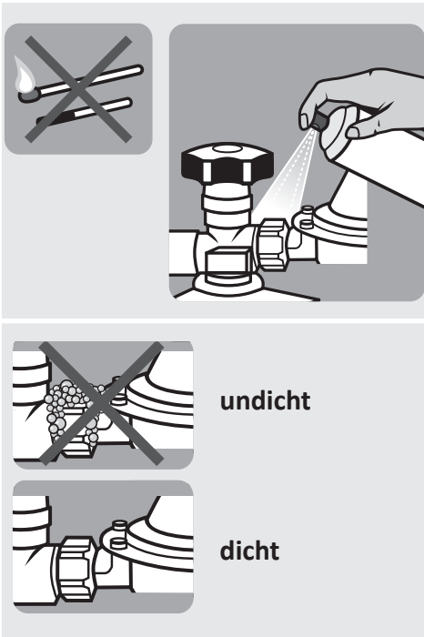
Abb.3: Dichtheitsprüfung
