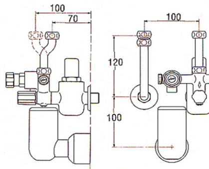
Strichzeichnung KV 40 - Art.-Nr. 166.13 Z02
