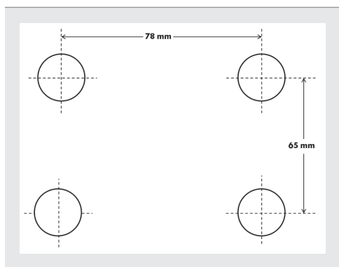
Abb.1: Bohrlöcher
