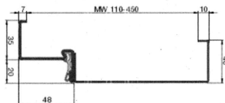
Eckzarge mit Ergänzungszarge
