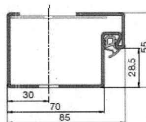
Blockzarge für den Einbau auf der Wand
