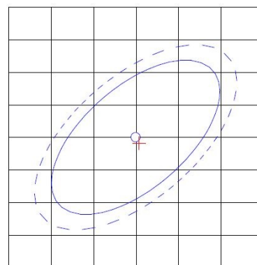
CIE1931色品图
